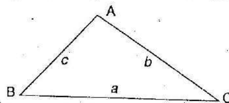
الشكل 99 - قانون جيب التمام. أنظر المداخل الرئيسية.
