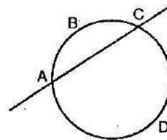
الشكل 19 - قوس. ABC القوس الأصغر و ADC القوس الأكبر
