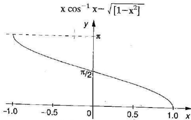
الشكل 23 - قوس جيب التمام.
