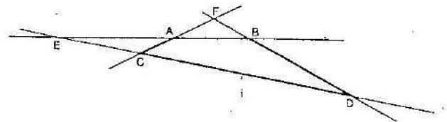
الشكل 76 - رباعي أضلاع تام. أنظر المدخل الرئيسي.
