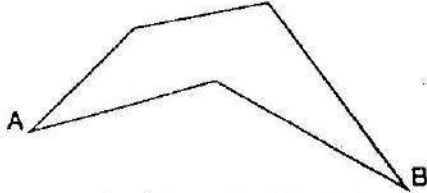
الشكل 79. مقعر. مضلع مقعر.
