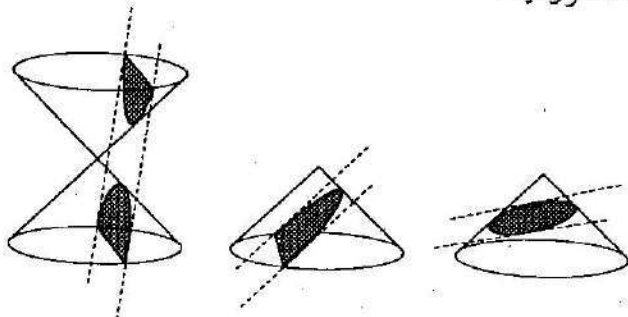
الشكل 82 - قطوع مخروطية. أنظر المدخل الرئيسي.
