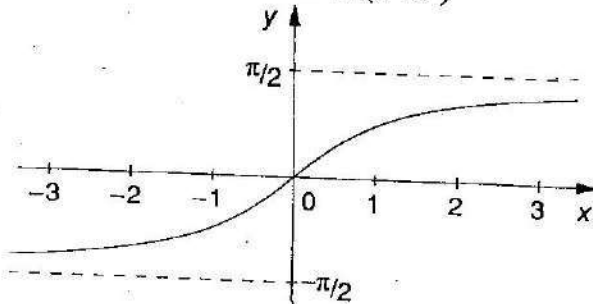
الشكل 31 - قوس الظل.
