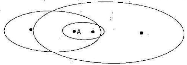
الشكل 85 - متحد البؤرة. A بؤرة للاهليلجات الثلاث.
