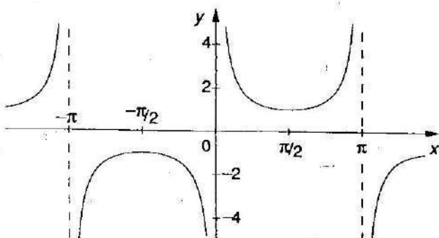
الشكل 95 - قاطع التمام. بيان دالة قاطع التمام
